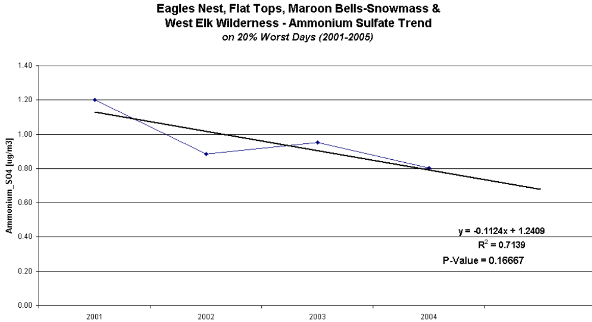
Figure G -1: Ammonium Sulfate Trend
